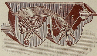
Coupe de la machine Kodak pour en montrer le mécanisme.
